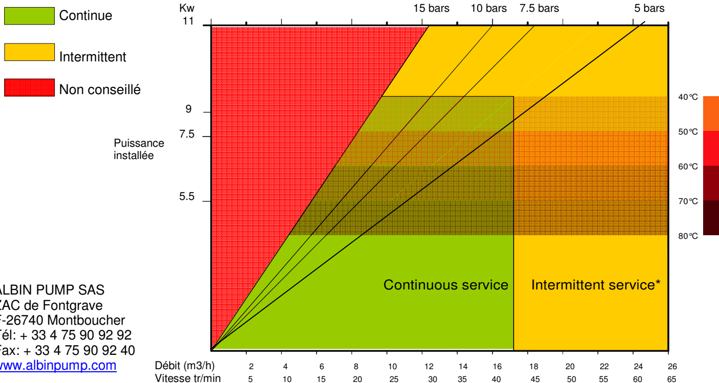
Pompe ALHX 65
