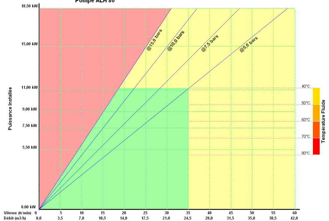
Pompe ALH 80
