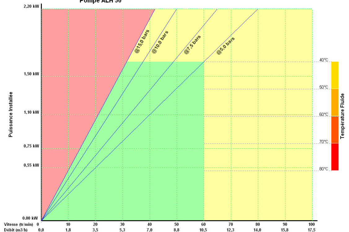
Pompe ALH 50
